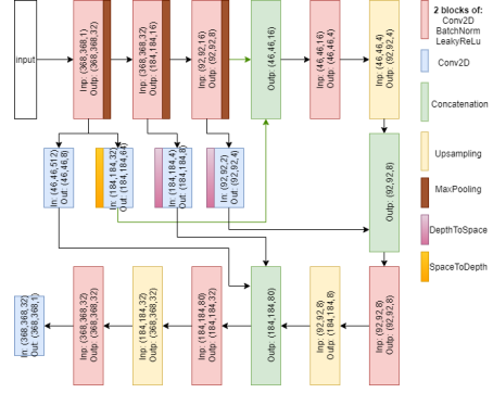
FIGURE 1 – Exemple d'architecture de réseau de neurones optimisée à l'issue d'une étape de recherche automatique, exploitable pour la reconstruction de cartes RSSI à partir de données expérimentales au sein de la ville de Grenoble.
