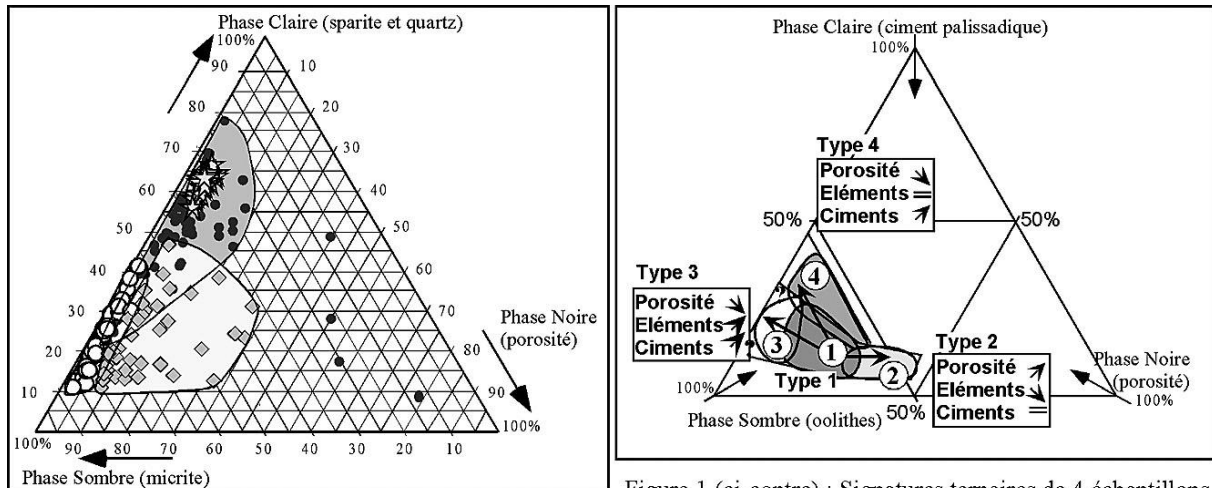
Figure 1 (ci-contre) : Signatures ternaires de 4 échantillons de la Formation du Calcaire grossier (200 mesures)
