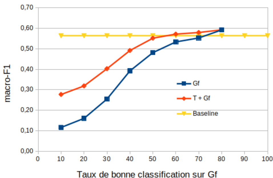
FIGURE 3 : Performances (macro-F1) en fonction de la qualité (taux de bonnes précisions en %) du classifieur servant au filtrage des données générées automatiquement ; données MediaEval avec la classifieur régression logistique.
