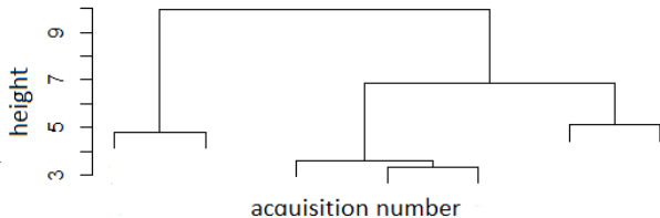
Fig. 4: Dendrogram
