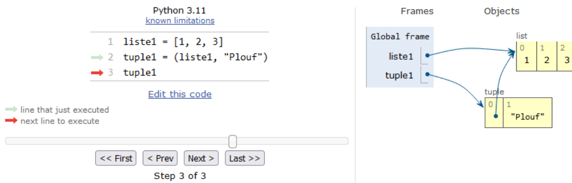
FIGURE 14.1 – Tuple contenant une liste.
