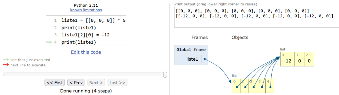
FIGURE 12.3 – Initialisation d'une liste de listes avec l'opérateur de duplication.
