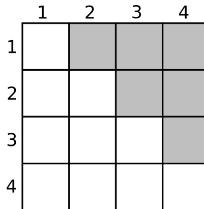
FIGURE 5.2 – Demi-matrice sans la diagonale (en gris).
