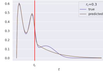
(d) r_c = 0.3, \tilde{p} = 3
