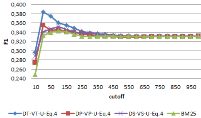
Figure 1. Impact de l'unité d'information considérée (S/P/T) dans l'estimation du modèle vital
