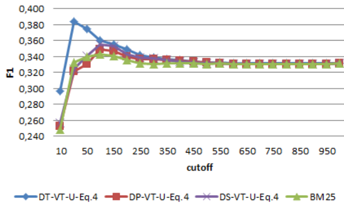
Figure 2. Impact de l'unité d'information considérée dans le document (S/P/T) dans l'évaluation de sa vitalité
