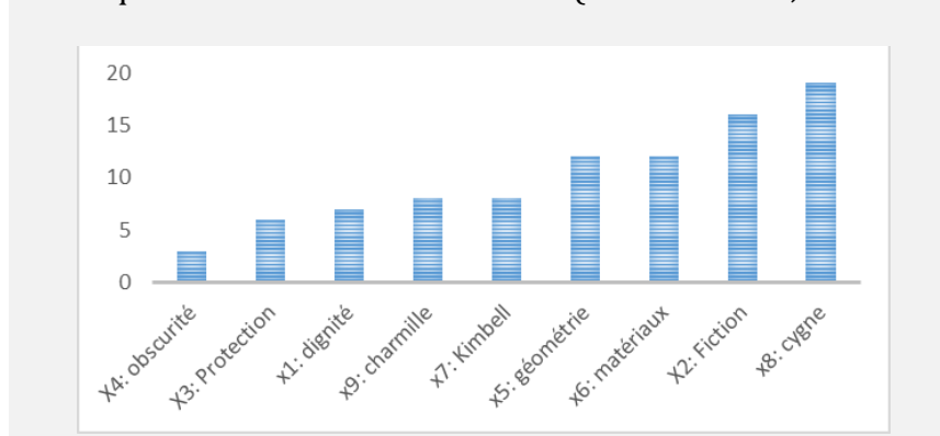
Figure 14 : mise en codimension des différents attracteurs
