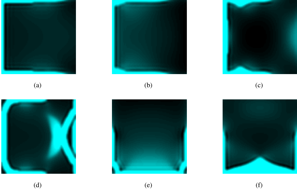
FIG. 5: Optimal topology for \bar{K} for the PZT/PVDF composite: (a) \bar{K}_{1111} ; (b) \bar{K}_{2211} ; (c) \bar{K}_{1212} ; (d) \bar{K}_{2222} ; (e) \bar{K}_{2212} ; (f) \bar{K}_{1211} .
