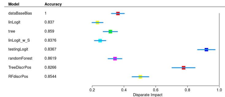
FIGURE 1 – Précision de la prévision (accuracy) et effet disproportionné estimé par un intervalle de confiance sur un échantillon test (taille 9000) pour différents modèles ou algorithmes d'apprentissage.
