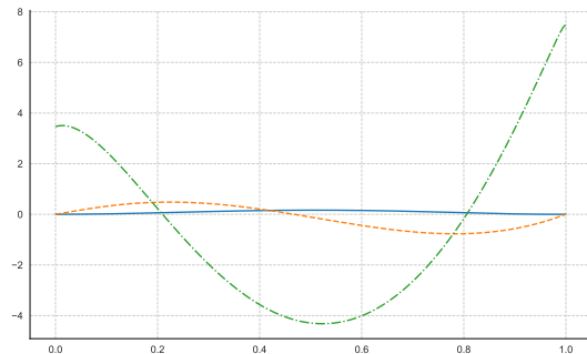
(d) CTIF with \gamma = 1/2 and \rho = -3
