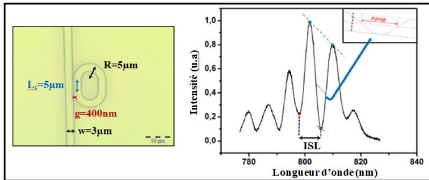
Fig. 2: Imagerie par microscopie optique d’une des familles de structures micro-résonateurs et son spectre associé et mesuré par analyseur de spectre optique. L_c représente ici une longueur de couplage guide/MR.
