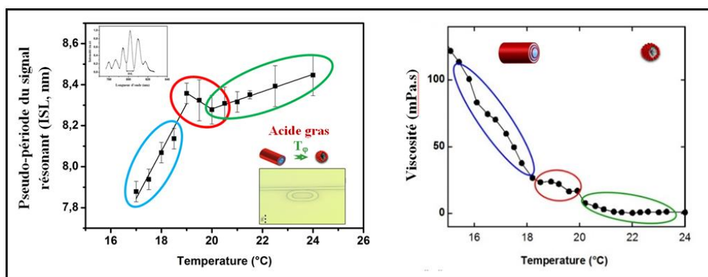
Fig. 4: Evolution du paramètre spectral 'pseudo-période' (ISL) du signal résonant du capteur lors de la dynamique de transition de phase de l'acide gras (acide 12-hydroxystéarique) ; modification de morphologie à l'échelle microscopique lors de la transition à T_{\phi} ( \mu -tubes \Rightarrow nano-micelles) corrélée à une variation/modification viscoélastique (mesures de rhéologie) à l'échelle macroscopique.
