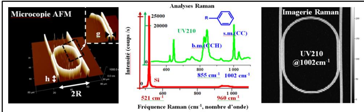
Fig. 1: Contrôle qualité du dispositif photonique. Microscopie à force atomique (AFM, rugosité de surface < 2 nm), analyses par spectroscopie Raman de surface et/ou de section des composants, imagerie Raman...
