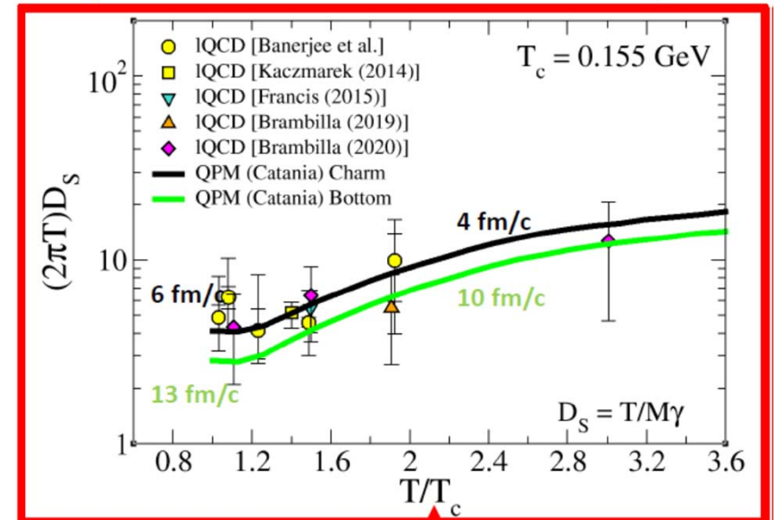
Spatial diffusion coefficient of bottom quark
