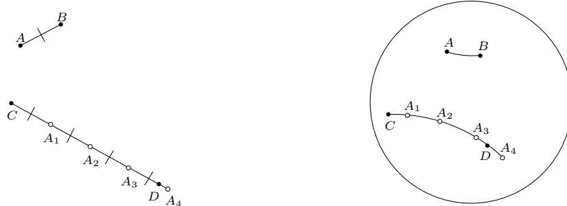
FIGURE 2 – Axiome d'Archimède
