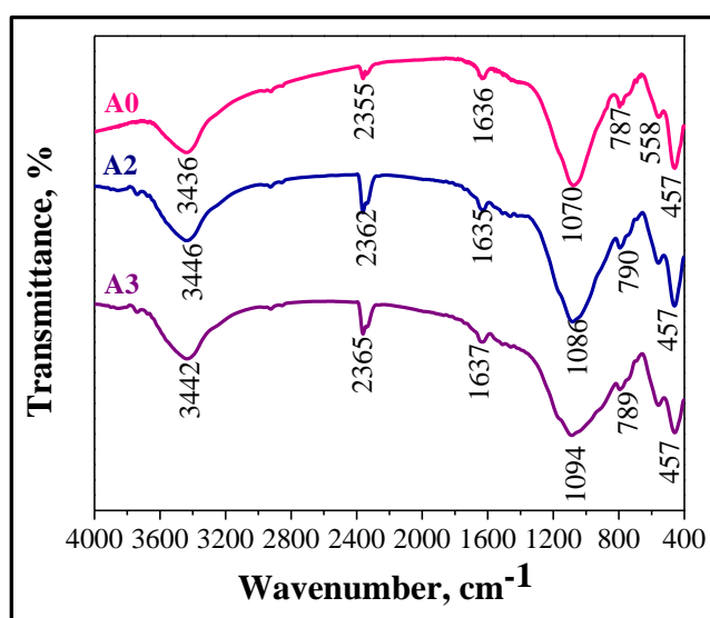
Figure 3a FTIR spectra for A0 vs. A2 vs. A3.
