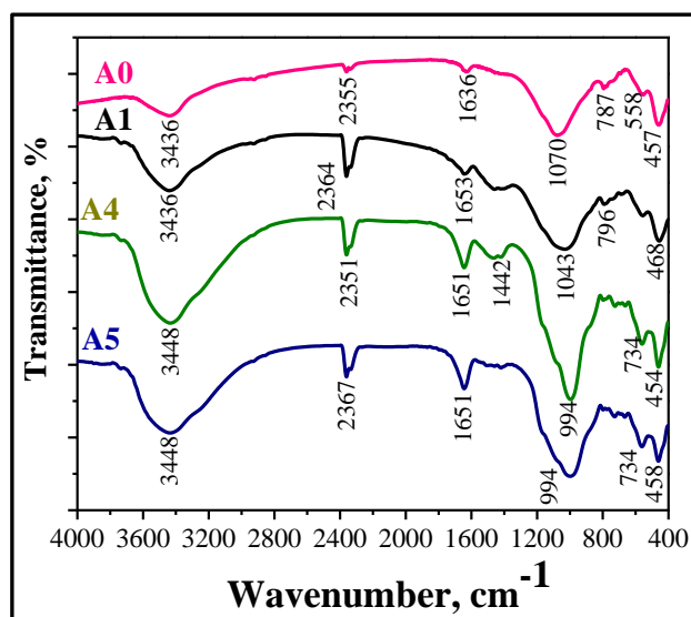
Figure 3b FTIR spectra for A0 vs. A1 vs. A4 vs. A5.
