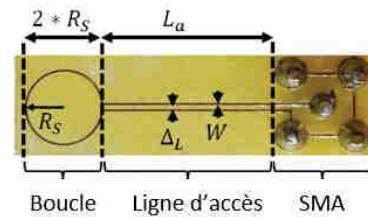
Fig. 1: Antenne intégrée
