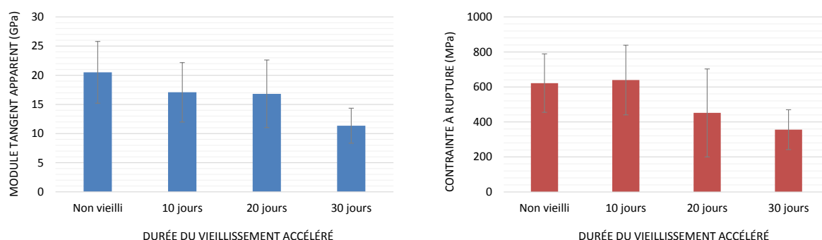
Fig.1 Evolution des propriétés mécaniques en traction des fibres de chanvre en fonction du temps de vieillissement accéléré
