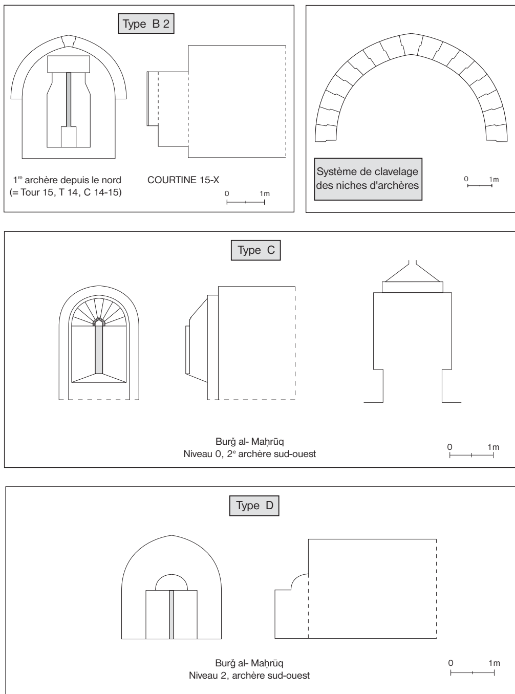
10. Typologie des archères.
