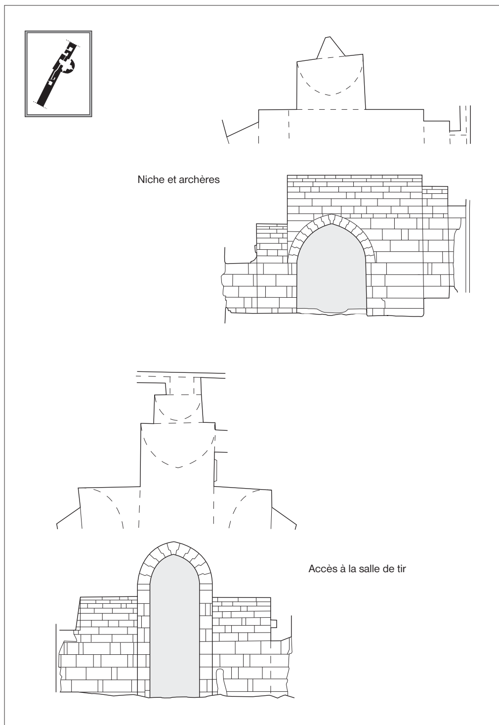
7. Tour 11, plans et élévations.
