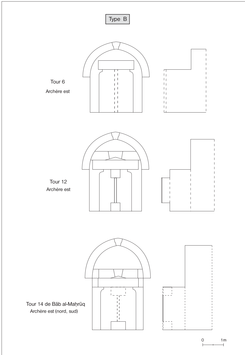
9. Typologie des archères.
