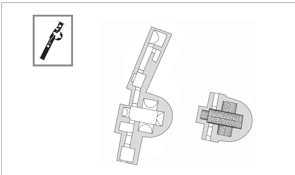
5. Plan et voûte de la tour 11.
