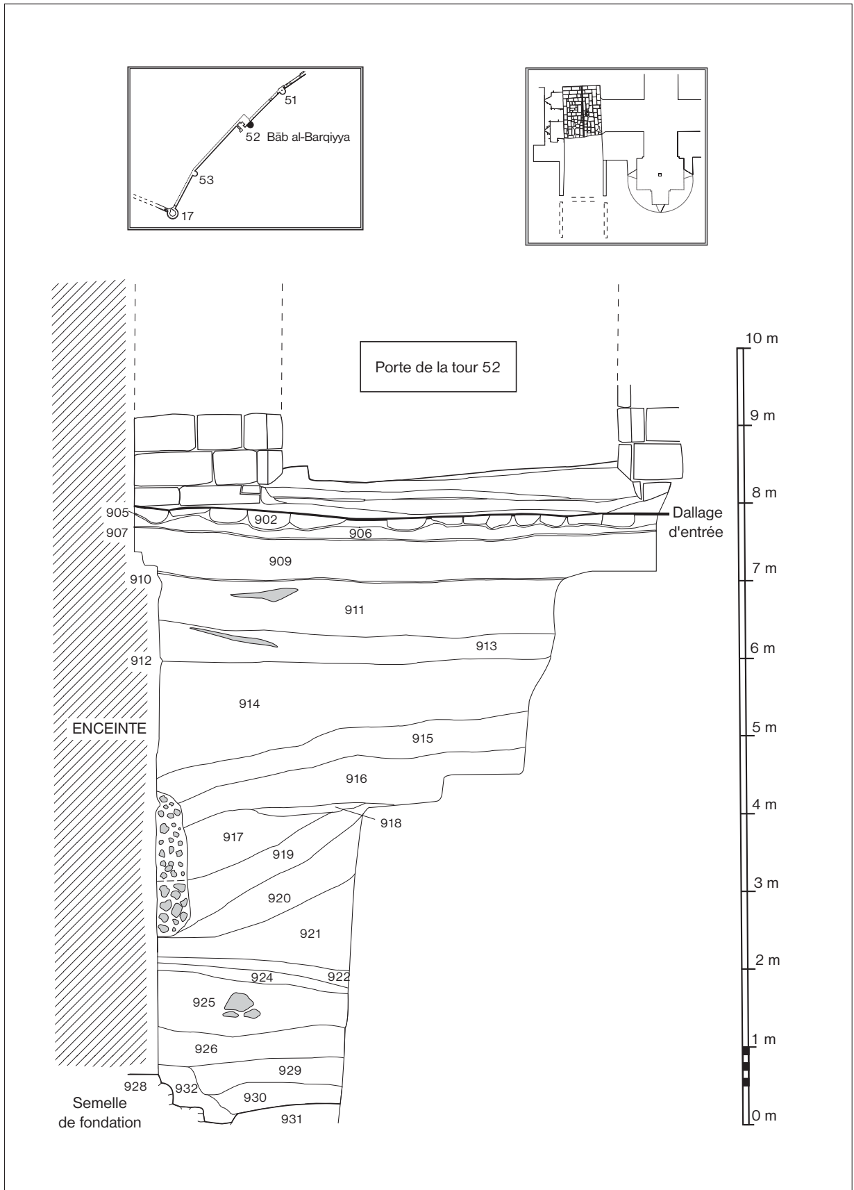
16. Coupe stratigraphique de Bāb al-Barqiyya.
