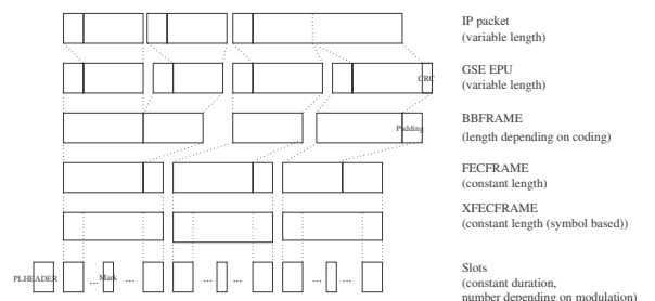
Fig. 1. DVB-S2/GSE encapsulation
