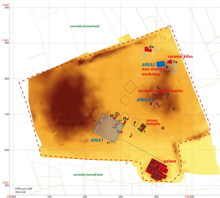
Figure 2. Layout of the Muweis site and excavated areas (© Musée du Louvre-Mission archéologique de Mouweis- Michel Baud, Marie Millet).
