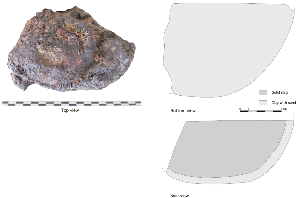
Figure 12. Solid slag MWS2002.27 (cl. N. Dieudonné-Glad, HeRMA, Université de Poitiers).
