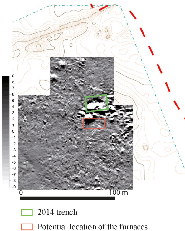
Figure 22. Hypothesis of the smelting furnaces location at Muweis in Area 2 (© Musée du Louvre-Mission archéologique de Mouweis- Yves Bière).
