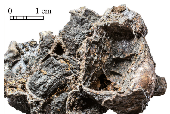
Figure 14. Slag MWS14-2000-S1C3.02 with charcoal prints and embedded charcoals (© Musée du Louvre-Mission archéologique de Mouweis-Hélène David-Cuny).
