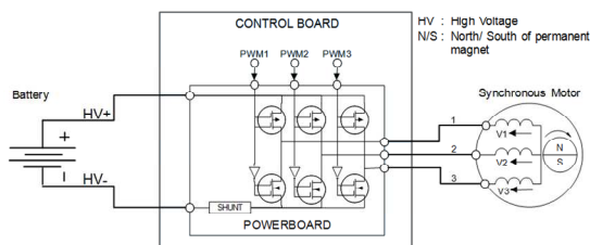
Figure 1: Schéma général de la chaîne de puissance modélisée
