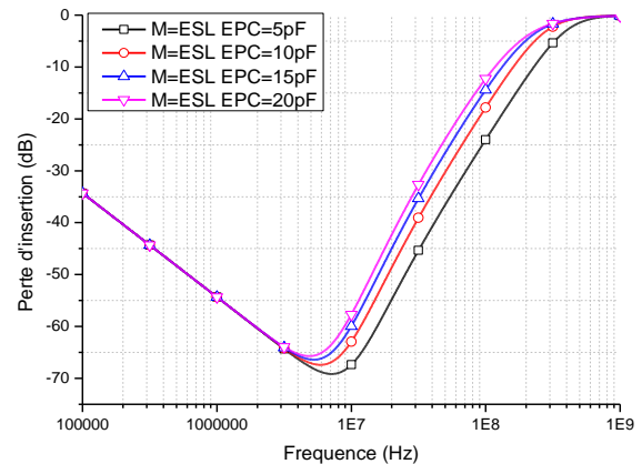
Figure 3 Perte d'insertion simulée d'un filtre LC optimisé ( M=ESL ) pour différentes capacités parasites (EPC) de la self
