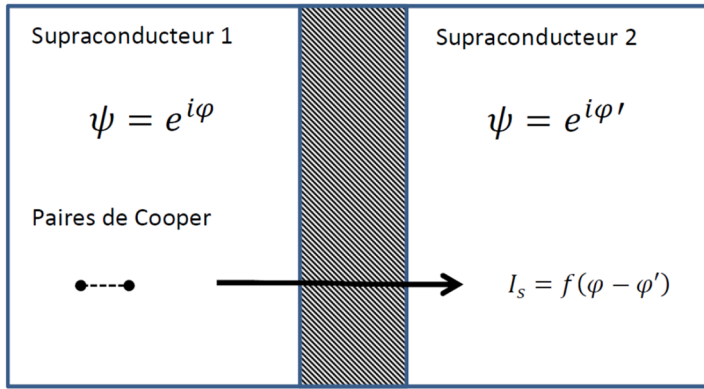
Figure 8 : Principe fonctionnel d'une jonction Josephson
