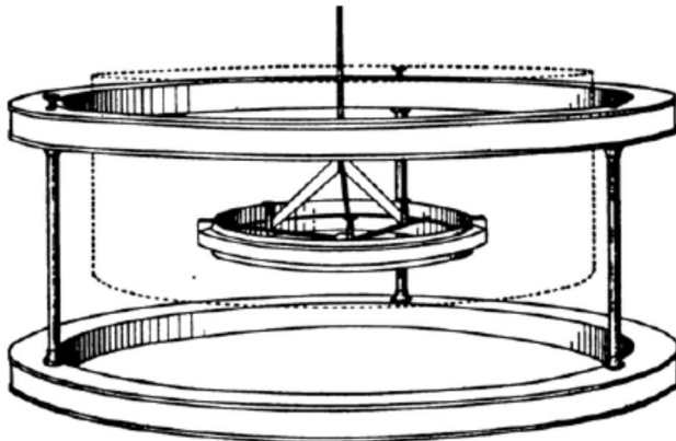
Figure 5 : Principe de la balance de l'Ampère
