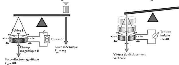
Figure 6 : Schéma de principe de la balance du Watt actuelle définie par Kibble
