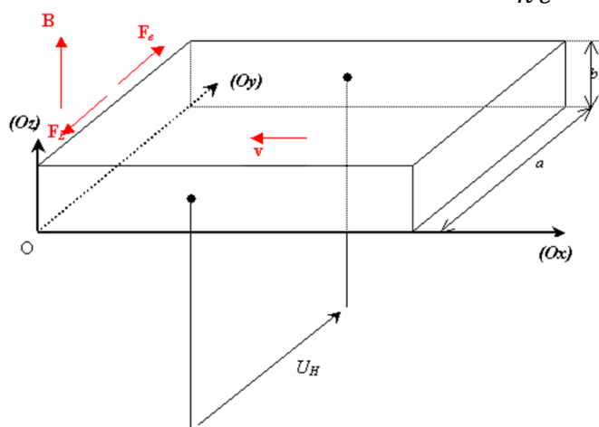
Figure 9 : Schéma de principe d'une cellule à effet Hall quantique
