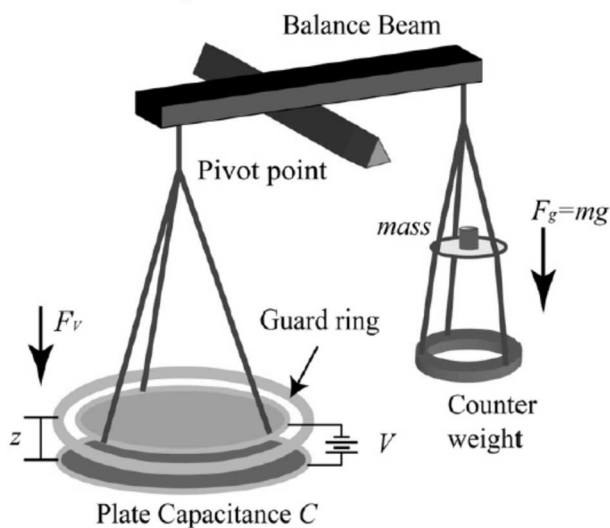
Figure 3 : Schéma de la balance du voltage absolu (extrait de l'article de R. Steiner 145 )
