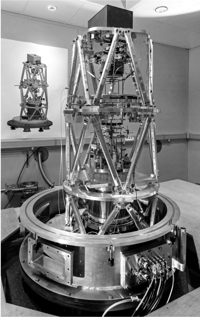
Figure 7 : La balance du Watt du BIPM en 2017 pendant une phase de maintenance
