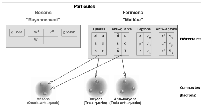
Figure 10 : Les différentes particules élémentaires selon le modèle standard
