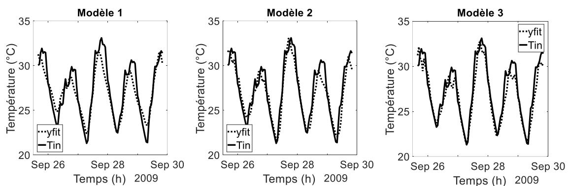
FIGURE 1. Comparaison entre la température intérieure observée (simulation) et estimée avec les modèles MLR 1, 2 et 3
