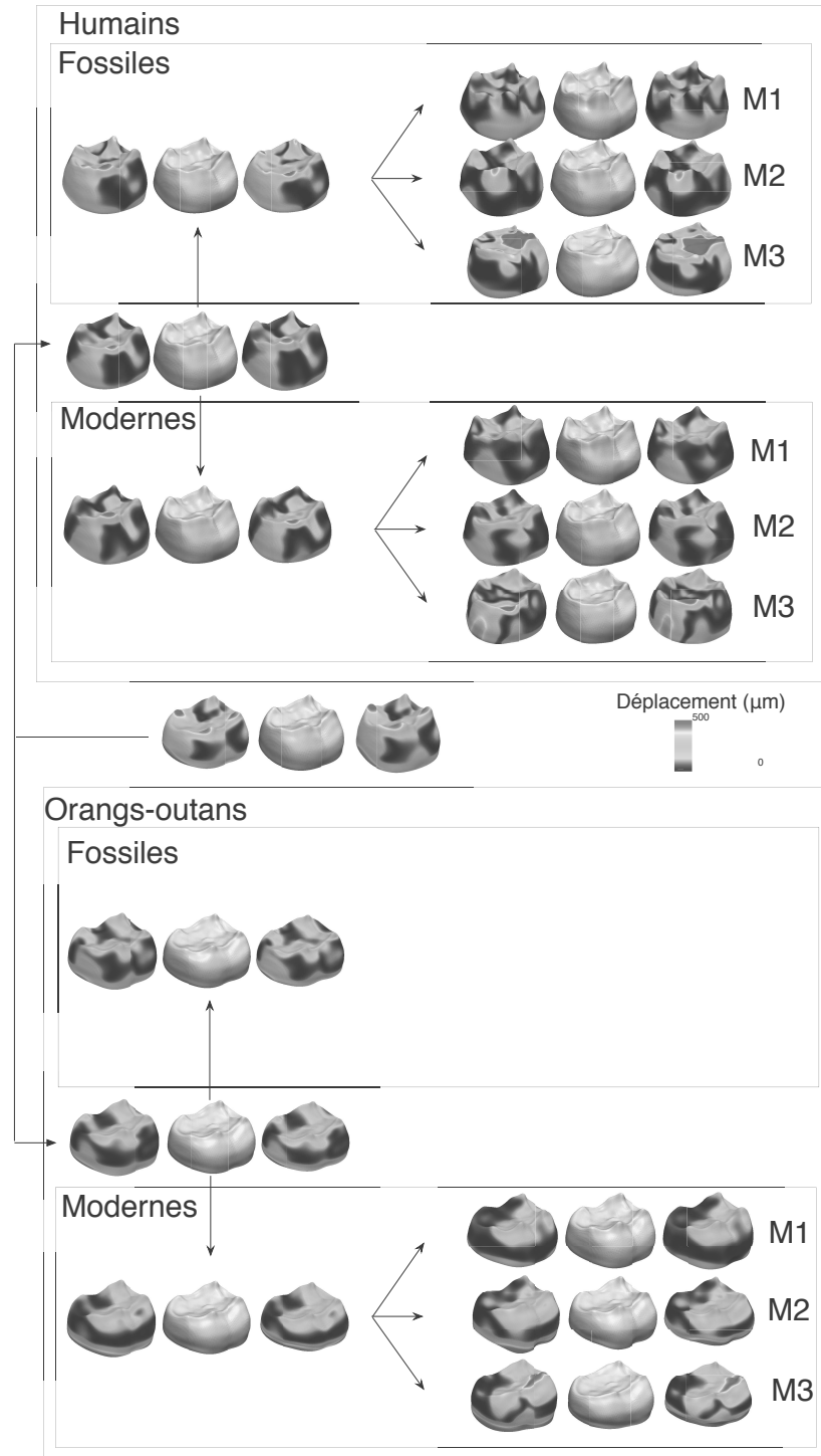
Figure 5: Représentation de la variabilité en fonction des catégories utilisées. Pour chaque catégorie, une forme moyenne a été générée, et la variabilité a été calculée en appliquant une analyse en composantes principales sur les vecteurs de déformation. Pour chaque sous-groupe, la valeur moyenne est représentée au centre, et les déformations à -\sigma (resp. +\sigma ) à gauche (resp. droite), selon le premier mode. Les couleurs sont relatives au déplacement cumulé en chaque point de la surface.
