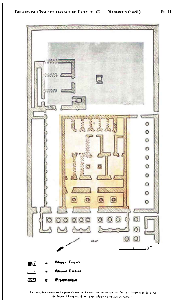
FIGURA 1. Las plataformas de Medamud según Bisson (Bisson de la Roque y Clere, 1928, vol. I).
