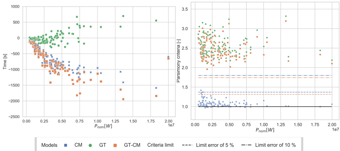
Figure 3: Différence en temps de simulation (gauche) et critère de parcimonie (droite) sur le NRMSE de la puissance fournie par le générateur, pour les modèles CM, GT et GT-CM
