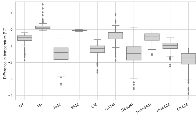
Figure 2: Impact des niveaux de détail des modèles sur la température de retour moyenne
