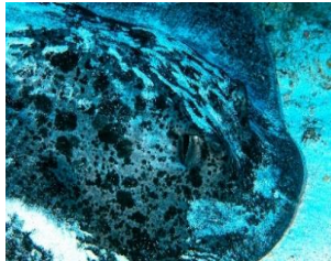
Taeniurops meyeri
