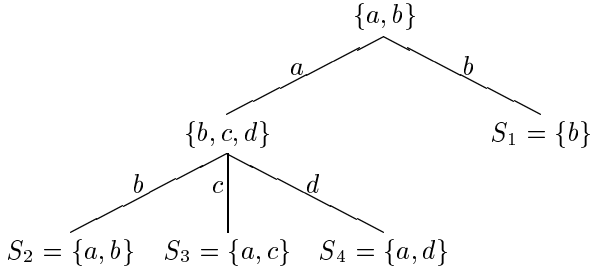
FIG. 1 – Calcul d'ensembles intersectants de \mathcal{C} = \{\{a, b\}, \{b, c, d\}\} selon [17]
