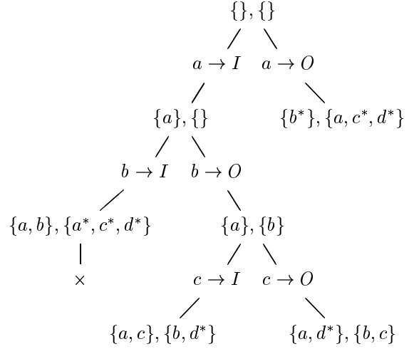
FIG. 2 – Arbre binaire de calcul des ensembles intersectants minimaux de \mathcal{C} = \{\{a, b\}, \{b, c, d\}\} : les nœuds sont représentés par les paires I, O correspondantes ; les éléments passés dans I et O à cause des propriétés de coupures sont indiqués par des astérisques. La croix indique une branche fermée car I(n) \cap O(n) \neq \emptyset .
