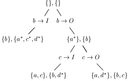
FIG. 3 – Arbre optimisé pour le calcul des ensembles intersectants minimaux de \mathcal{C} = \{\{a, b\}, \{b, c, d\}\} .
