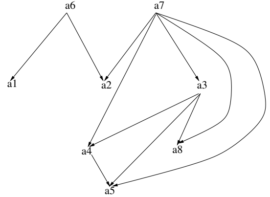
FIG. 4 – Graphe de la relation < obtenue à partir de l'exemple 2
