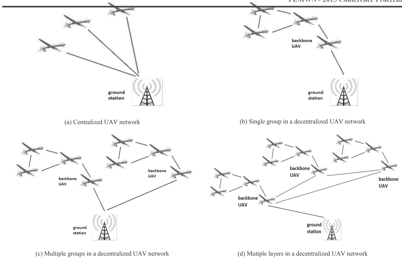
Fig.1. UAV topologies
