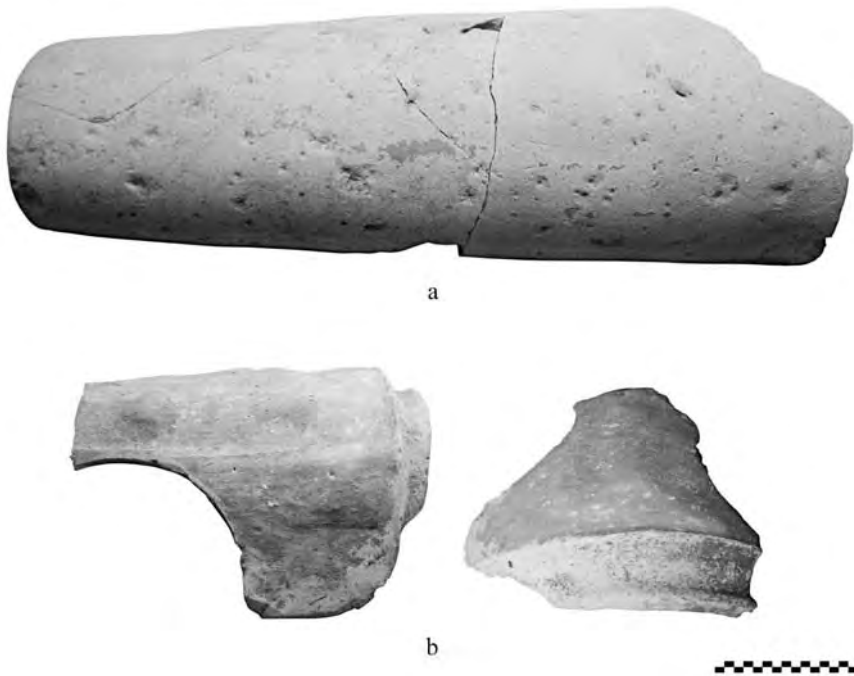
Fig. 2 a. Coprigiunto semicircolare; b. Coppo di colmo con resti di colore rosso
