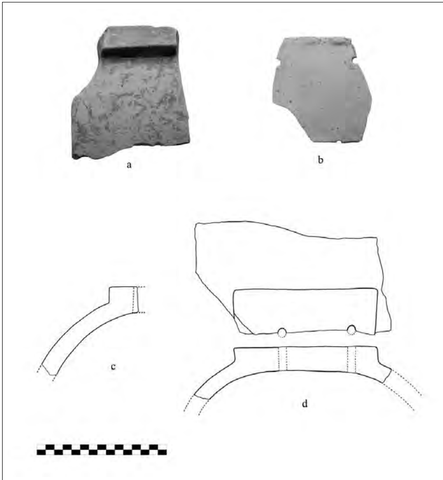
Fig. 5. Frammenti di coppi-plinto per statue acroteriali dall'ambiente 3
