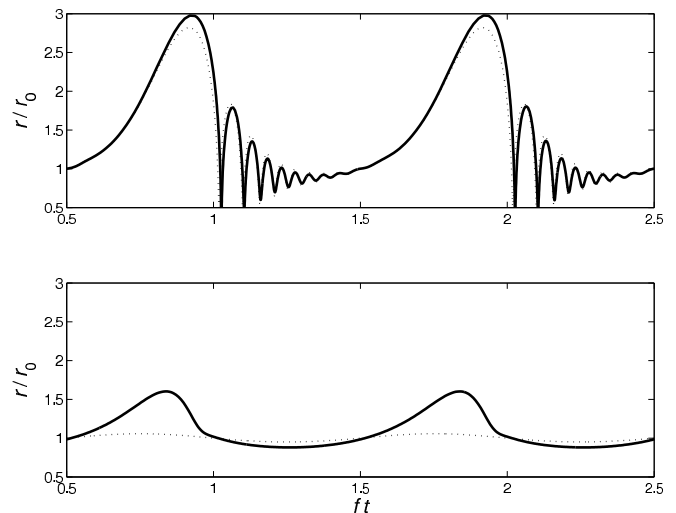
Abbildung 2: Berechnete Lösungen der angepassten Rayleigh-Plesset-Gleichung (punktierter Linie) und der angepassten Herring-Gleichung (fette Linie) mit c = 1480 \text{ ms}^{-1} , \frac{\omega}{2\pi} = f = 0,5 \text{ MHz} , p_0 = 1 \text{ atm} , p^+ = 210 \text{ kPa} , r_0 = 0,75 \mu\text{m} , \epsilon = 20 \text{ nm} , \mu = 10^{-3} \text{ Pa s} , \rho = 998 \text{ kg m}^{-3} und \sigma = 0,072 \text{ N m}^{-1} . Der obere Rahmen zeigt r-t -Kurven einer freien Gasblase, wobei S_f = 0 \text{ kg s}^{-1} , \delta_t = 0 , \mu_s = 10^{-3} \text{ Pa s} und \chi = 0 \text{ kg s}^{-2} . Der untere Rahmen zeigt r-t -Kurven einer hüllenstabilisierten Mikroblase mit S_f = 0 \text{ kg s}^{-1} , \delta_t = 0 , \mu_s = 10^{-1} \text{ Pa s} und \chi = \frac{1,1}{8\pi} \text{ kg s}^{-2} .
