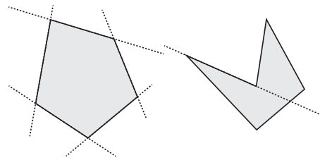
Figure 6. Seul le polygone de gauche est convexe.
