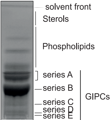
Os-GIPC (rice)
