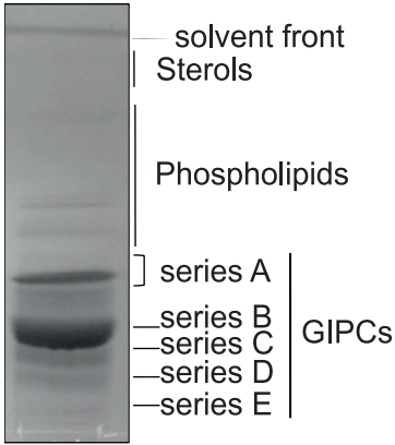
Ap-GIPC (leek)
