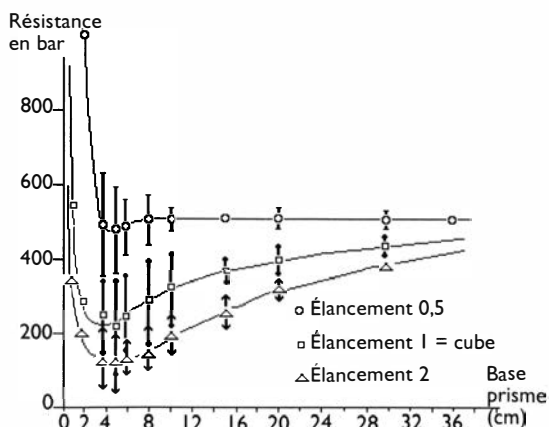
Figure 7 : Influence de la dimension de l'éprouvette sur la résistance mécanique du sel gemme (Mandzic)
