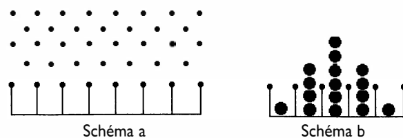
Figure 5 : L'expérience de Galton
