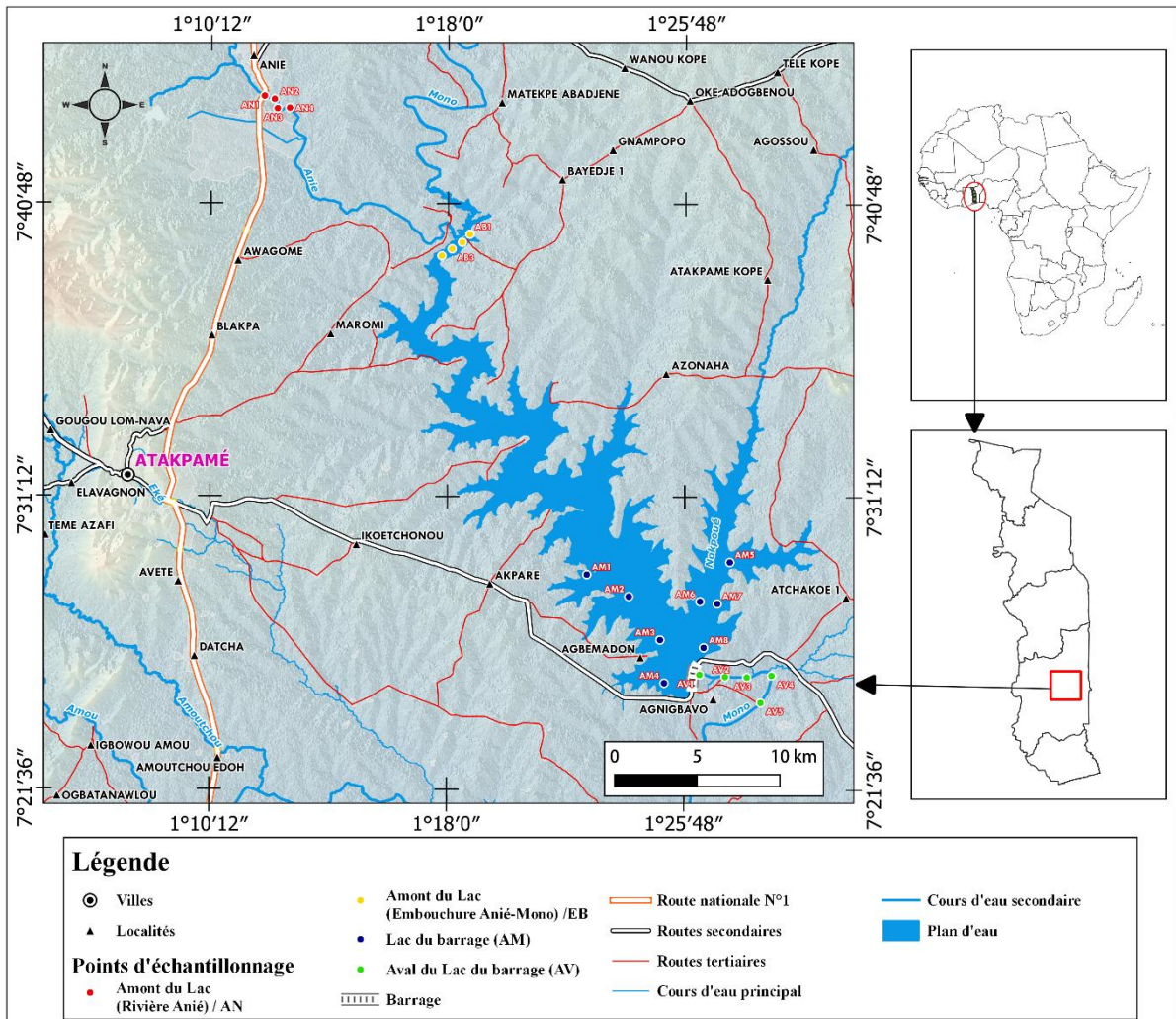
82 Figure 1 : Carte de la zone d'étude montrant les sites de prélèvements des sédiments.
