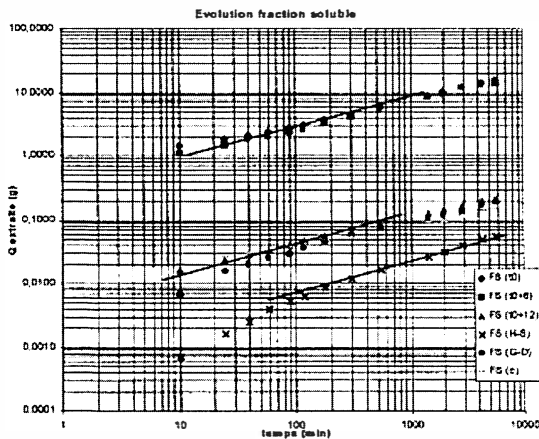
Figure 2 : Évolution de FS pour le déchet 3 pour les différents états de l'éprouvette
