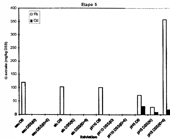
Figure 3 : Quantités de Pb et Cd extraites au cours des lixiviations de l'étape 5 (rapporté en mg/kg de déchet stabilisé) - déchet 3
