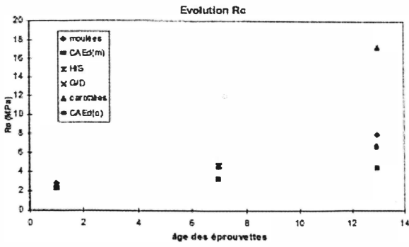
Figure 1 : Évolution de Re pour le déchet 1 pour les différents états de l'éprouvette
