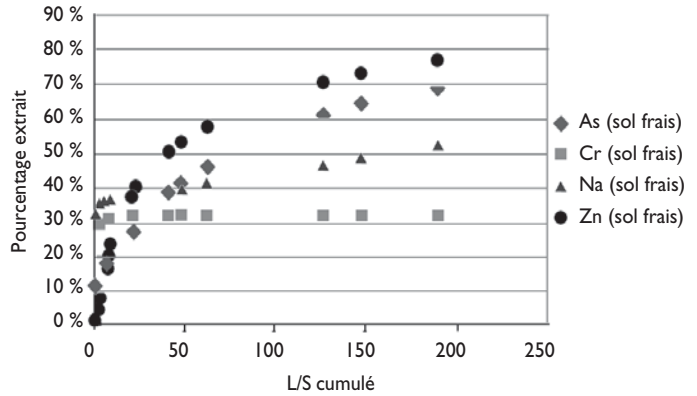
Figure 3: Pourcentages de polluants extraits (colonne sol frais)
