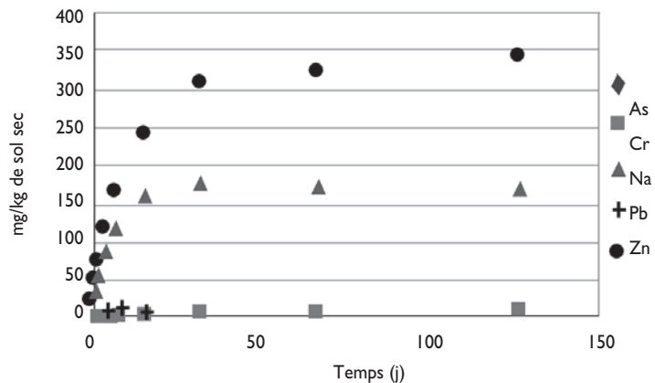
Figure 6: Relargage cumulé en mg/kg sol sec (CGLT sol réel pollué)
