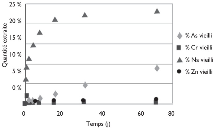
Figure 4: Pourcentages de polluants extraits (CGLT sol vieilli)
