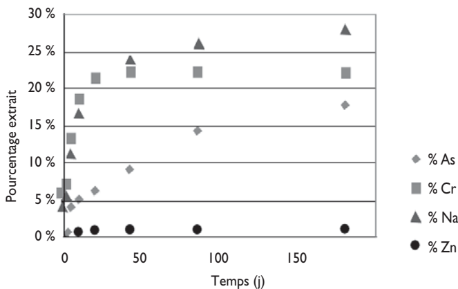
Figure 2: Pourcentages de polluants extraits (CGLT sol frais)
