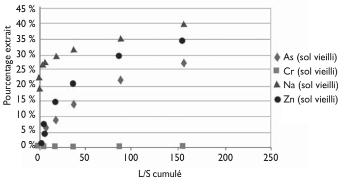
Figure 5: Pourcentages de polluants extraits (colonne sol vieilli)
