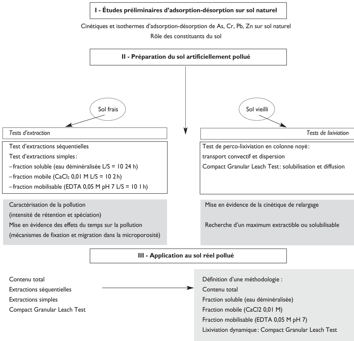
Figure 8 : Tableau synoptique, méthodologie expérimentale
