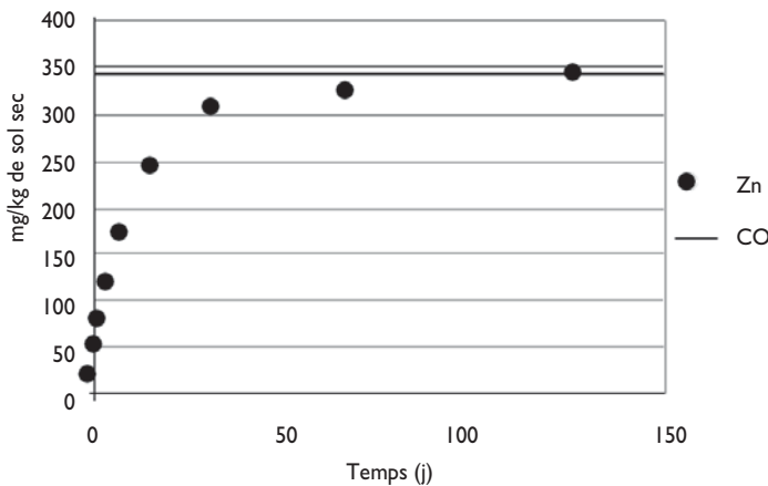
Figure 7: Relargage cumulé du zinc en mg/kg de sol sec (CGLT sur sol réel)
