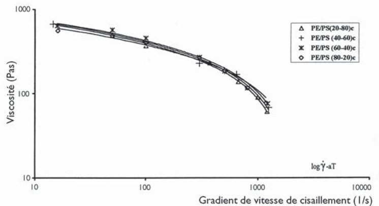
Figure 9 : Courbes maîtresses des mélanges PE/PS compatibles à 230°C
