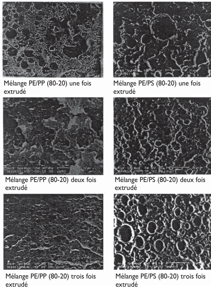
Figure 1 : Micrographies des surfaces après rupture pour les mélanges PE/PP et PE/PS de composition 80/20 ayant subi différents nombres d'extrusions. X 978
