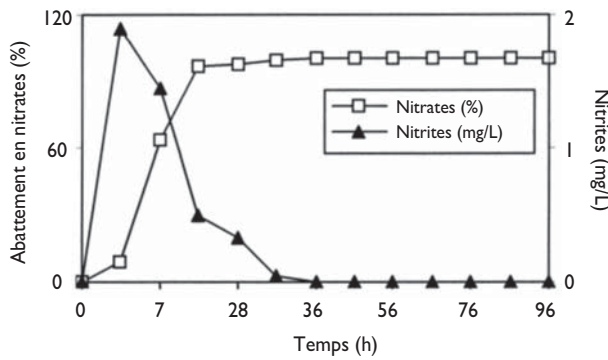
Figure 2 : Évolution des nitrites produits et de l'abattement en nitrates durant l'essai 1
