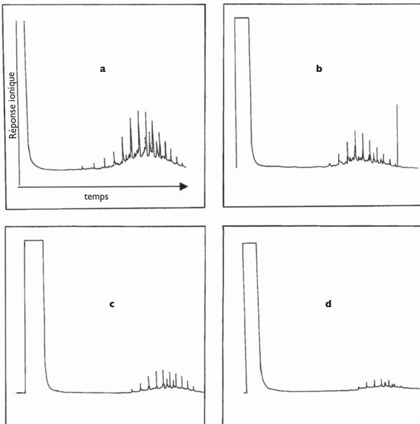
Figure 1 : Spectres des prélèvements à l'état initial (a), après 24 h (b), 48 h (c) et 72 h (d).
