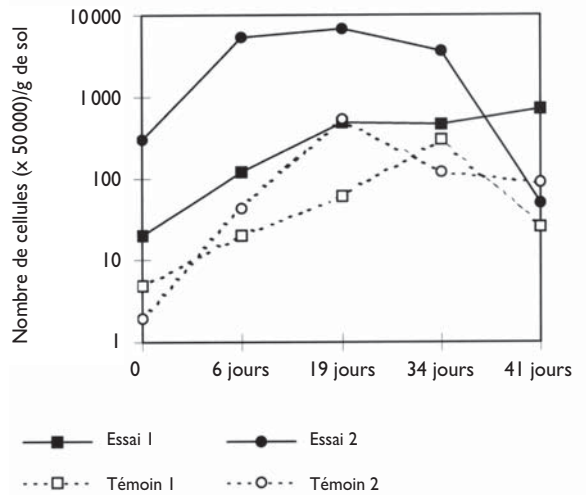
Figure 7 : Dénombrement de la population bactérienne adaptée aux hydrocarbures des bacs de sable grossier.
