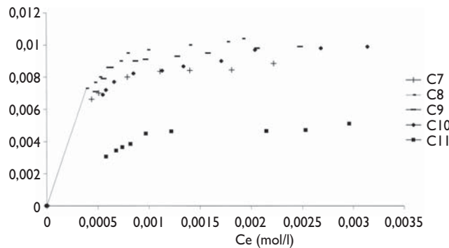
Figure 1b : Isothermes d'adsorption de l'iode par les charbons actifs commerciaux
