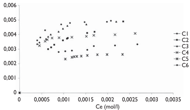
Figure 1a : Isothermes d'adsorption de l'iode par les charbons de rafles
