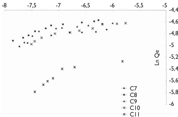
Figure 3b : Transformées linéaires de Freundlich (charbons commerciaux)
