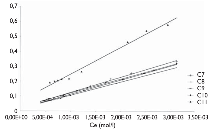
Figure 2b : Transformées linéaires de Langmuir (charbons commerciaux)
