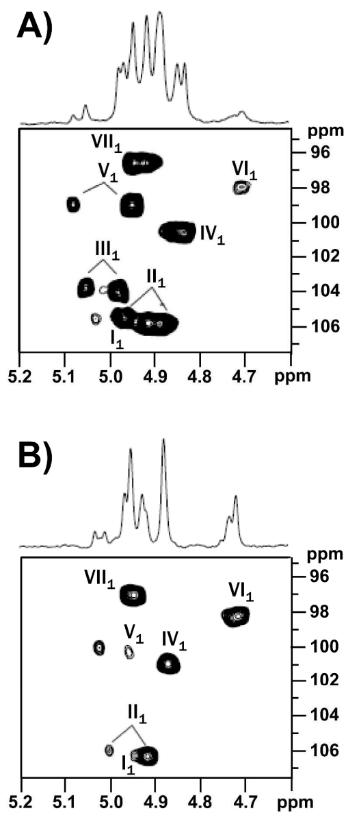
Figure 6: 2D ^1\text{H} - ^{13}\text{C} HMQC NMR spectra expansion ( \delta^1\text{H} : 4.60-5.15 and ^{13}\text{C} : 97.0- 113.0) of M. smegmatis LAM (A) and compound X (B) in \text{D}_2\text{O} at 298K. I : 3,5- \alpha -Araf ; II : 5- \alpha -Araf ; III : 2- \alpha -Araf ; IV : t- \alpha -Manp ; V : t- \beta -Araf ; VI : 6- \alpha -Manp ; VII : 2,6- \alpha -Manp.
