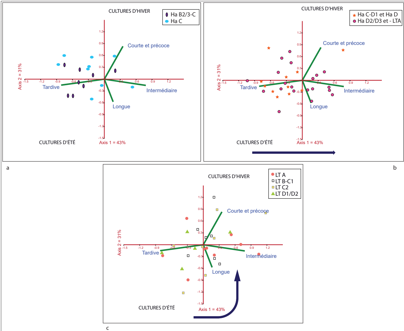
Fig. 14. Saison préférentielle des semis. ACC sur 77 sites, 77 taxons (adventices strictes) et 4 attributs. L'axe 1 détermine 43 % de la variance. a. Sites des 8 e -7 e siècles a.C. ; b. Sites des 7 e -5 e siècles a.C. ; c. Sites des 5 e -1 er siècles a.C. (DAO V. Zech-Matterne, CNRS).
