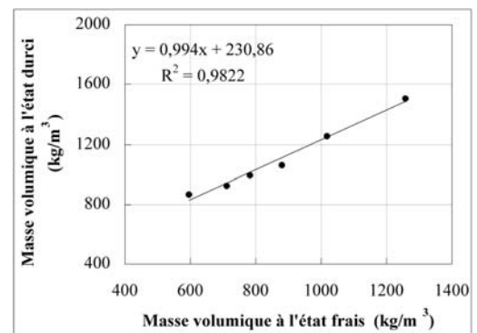
Figure 5. Relation entre les masses volumiques du composite CCCC à l'état frais et à l'état durci.
