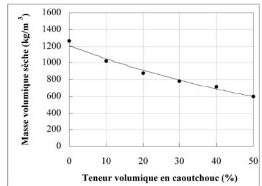
Figure 4. Evolution de la masse volumique sèche du composite CCCC en fonction de la teneur en caoutchouc.
