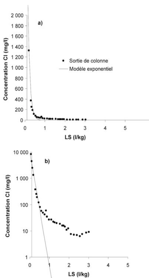
Figure 3 : Tentative de reproduction des concentrations en chlorures de la grande colonne (bas de la colonne) à l'aide du modèle de décroissance exponentielle.
