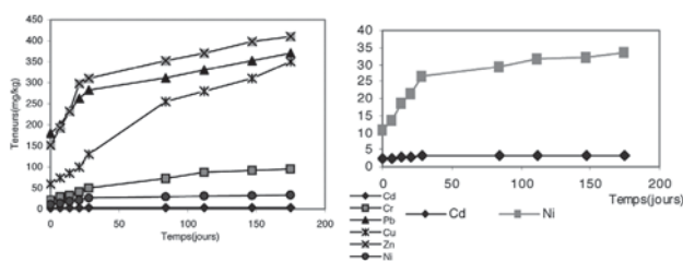
Figure 3 : Evolution des teneurs en métaux lourds durant le processus du compostage au sein de l'andain DTS
