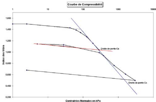
Figure V. Courbe de compressibilité des sédiments pollués
