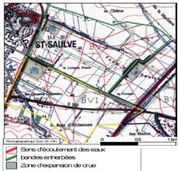
Figure 5 : Proposition théorique d'aménagement pour lutter contre les transferts de sédiments, réguler les débits et montrant la disposition d'un réseau éventuel.
