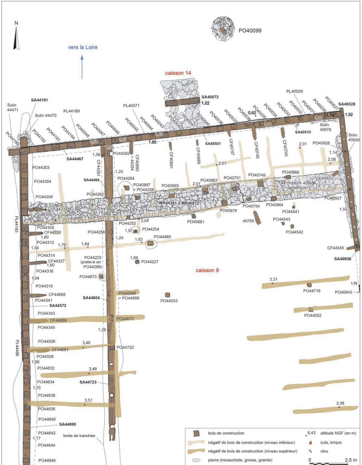
Fig. 5 – Plan du grand caisson n° 9 et de sa charpente en bois (DAO: J. Mouchard, M. Yacger).
